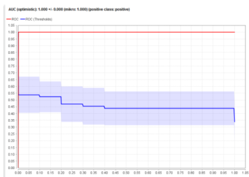
Gambar 4. Kurva ROC k-NN
