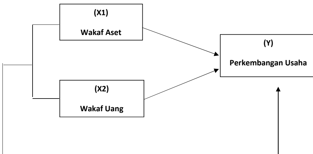
Gambar 1. Kerangka Teoritis
